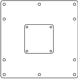
(1)Adaptor plate-a
